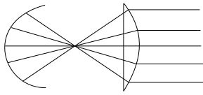
Plankonvex/Stufenlinse (Kugelspiegel)
