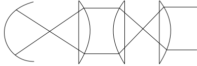
Profilier mit Vario-Optik (Kugelspiegel)
