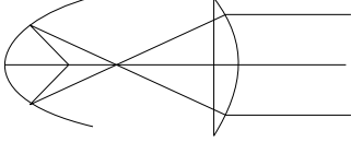
Profilier mit Festoptik (Ellipsenspiegel)
