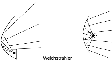
Weichstrahler
